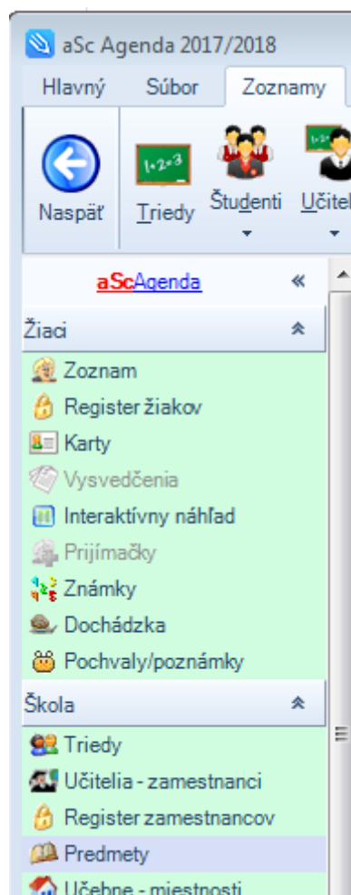
Obrázok 15 - Predmety
