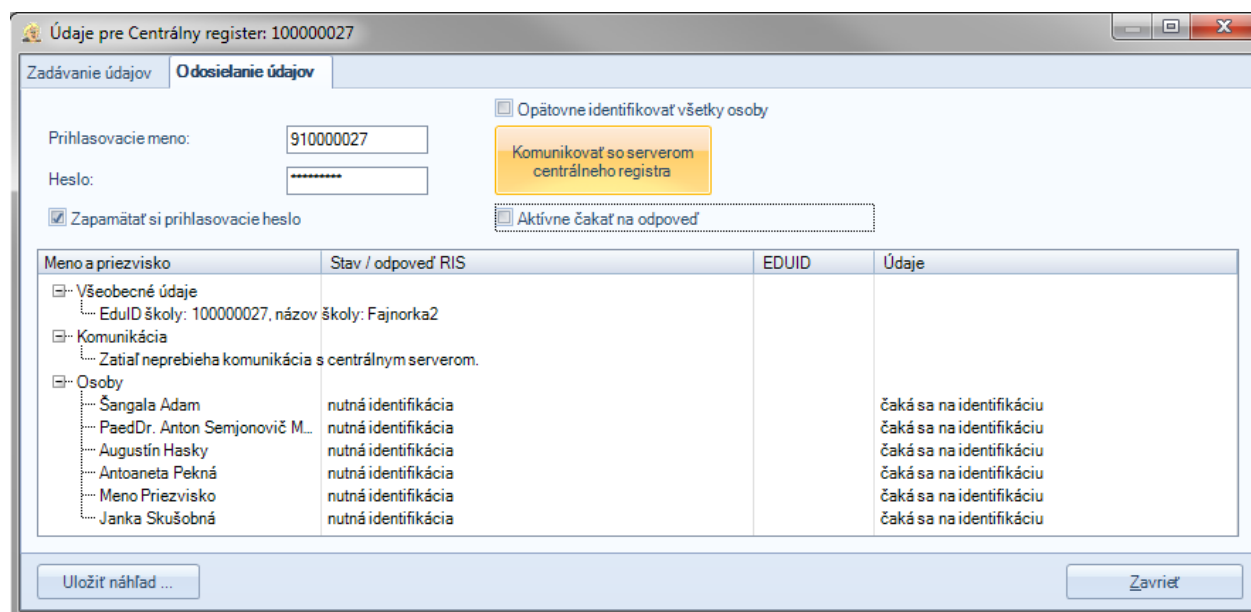
Obrázok 45 - Odosielanie údajov
