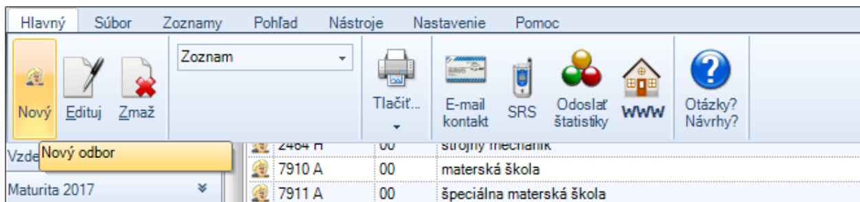
Obrázok 8 - Nový odbor
