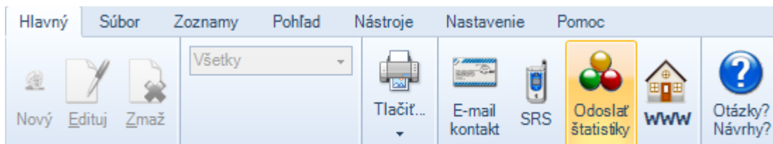
Obrázok 42 - Odoslať štatistiky
