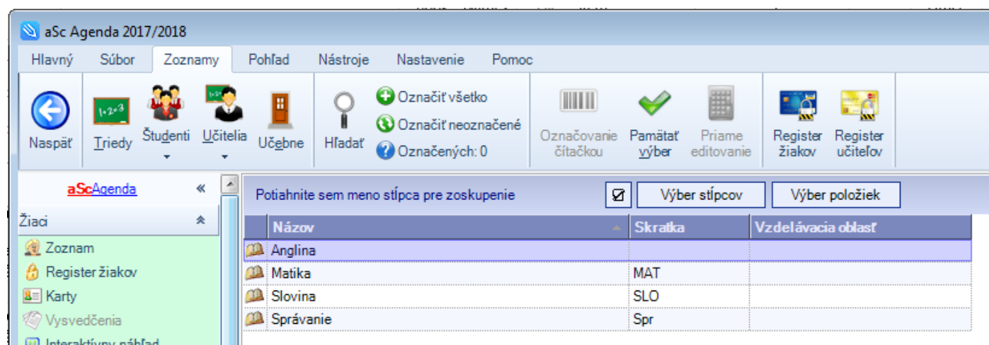
Obrázok 16 - Zoznam predmetov
