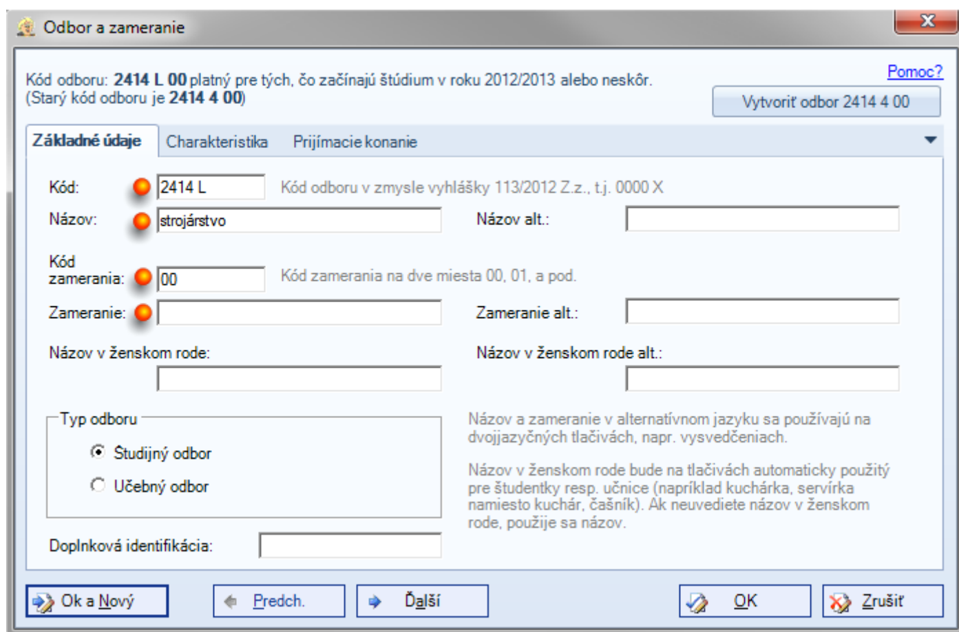
Obrázok 10 - Pridávanie ŠaUO
