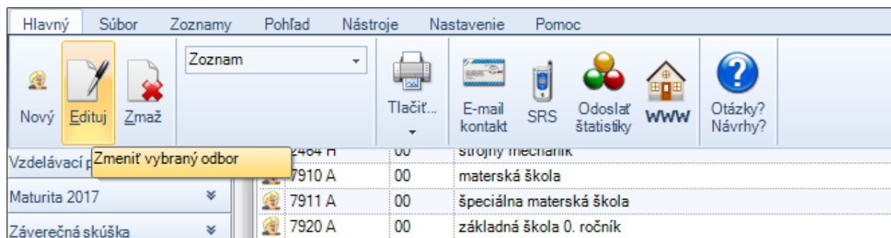
Obrázok 9 - Editovanie odboru
