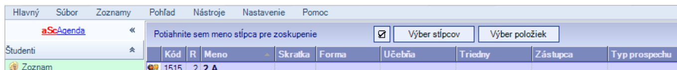
Obrázok 12 - Zoznam tried
