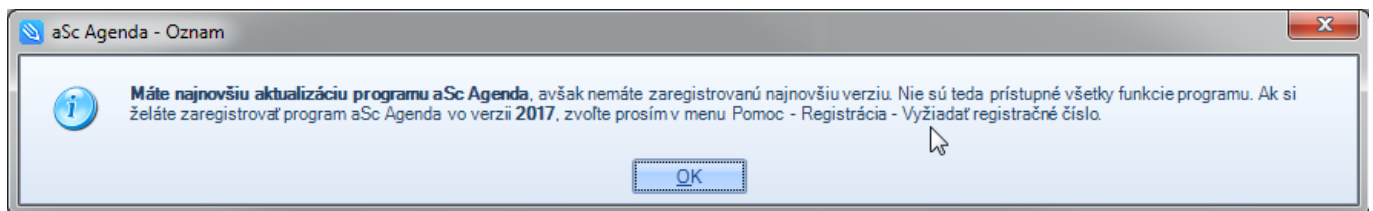
Obrázok 2 - Informačné okno
