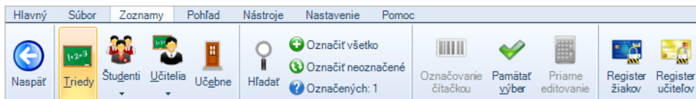
Obrázok 11 - Triedy
