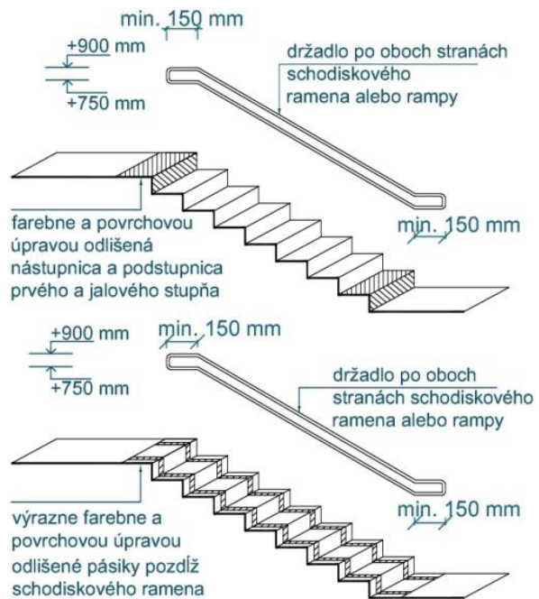
Riešenie schodiskového ramena s držadlami
