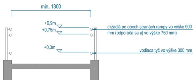
Priečný rez rampou (šírka ramena a osadenie držiadiel)
