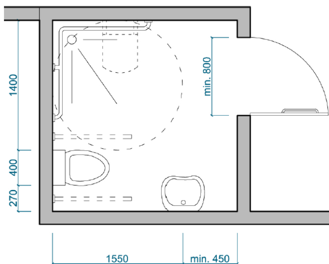
Minimálne rozmery bezbariérovej kúpeľne
