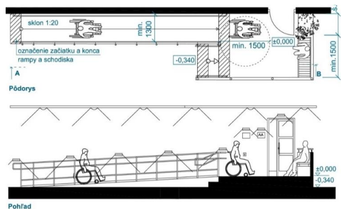
Riešenie rampy s optimálnym sklonom 1:20 pri výške 340 mm s dĺžkou ramena 6800 mm
