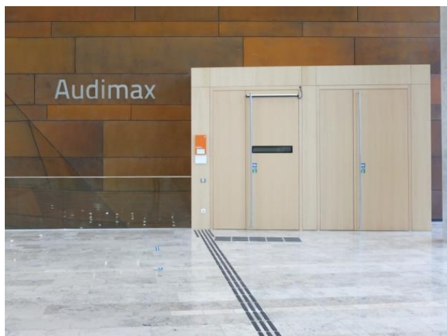
Príklad riešenia vstupnej haly s umelými vodiacimi líniami k sále (Ekonomická univerzita WU vo Viedni)
