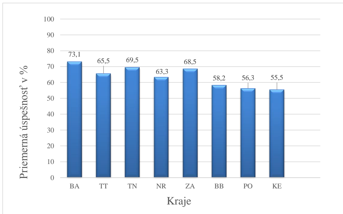
Graf č. 1.1 Priemerná úspešnosť podľa kraja v teste z matematiky
